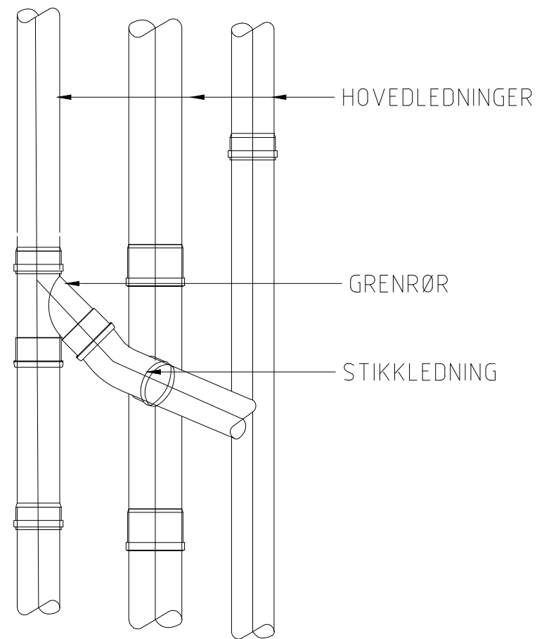
PLAN DIM. 150 - 300 mm
