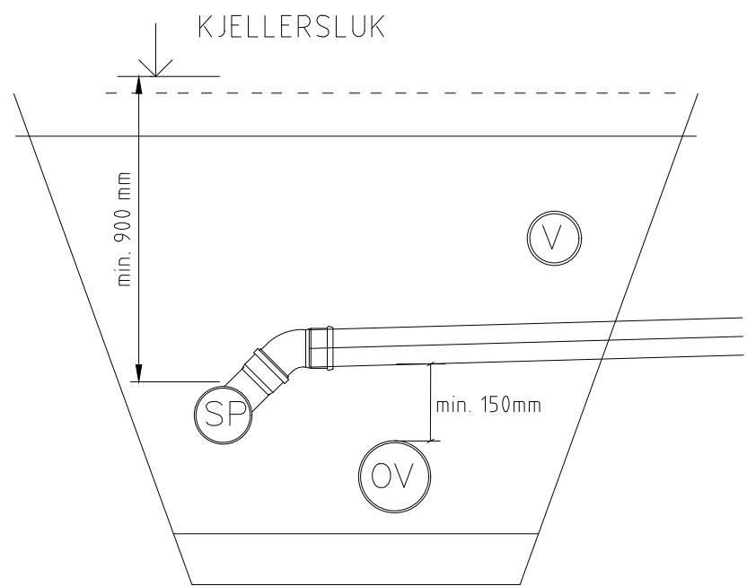
GRØFTESNITT
