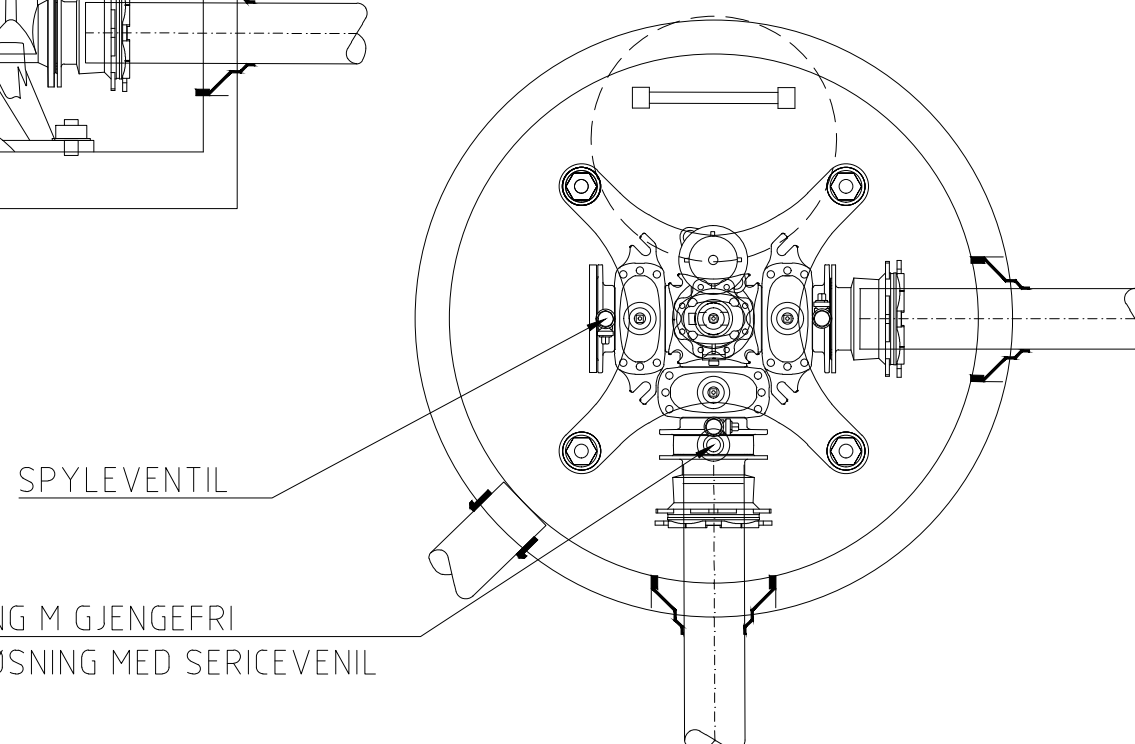
SNITT
