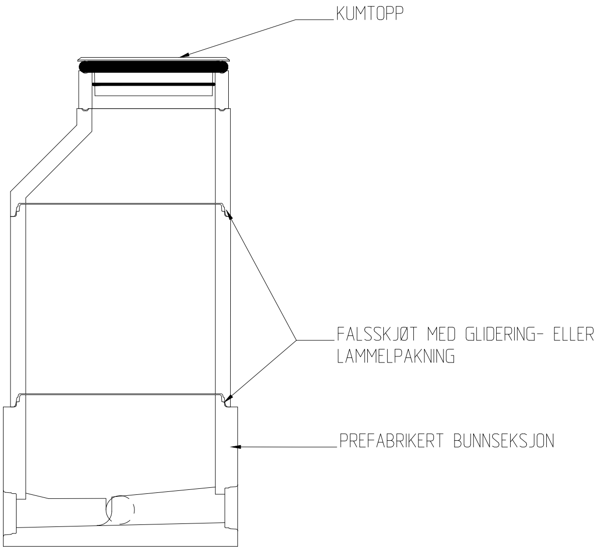
SNITT
