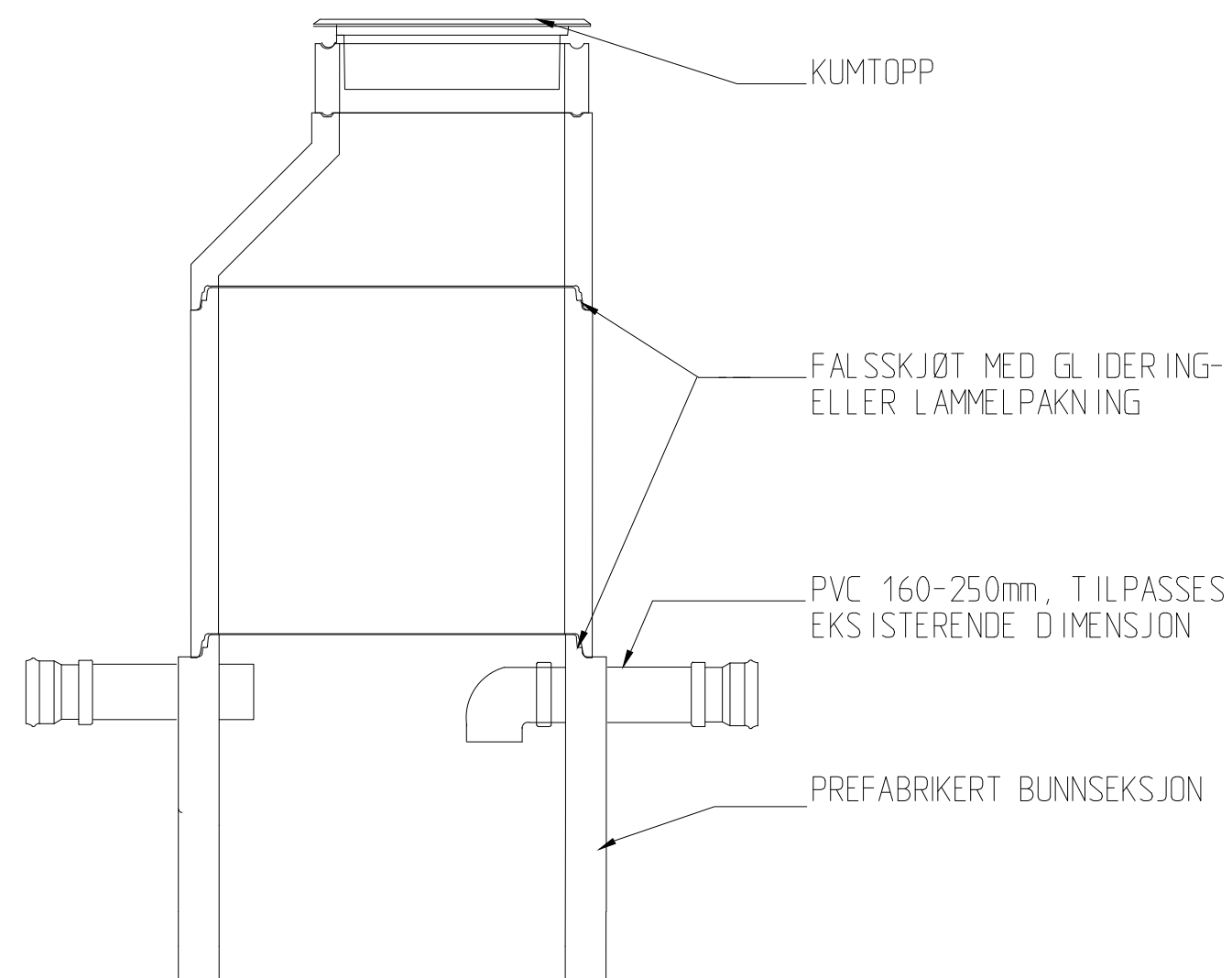
SNITT
