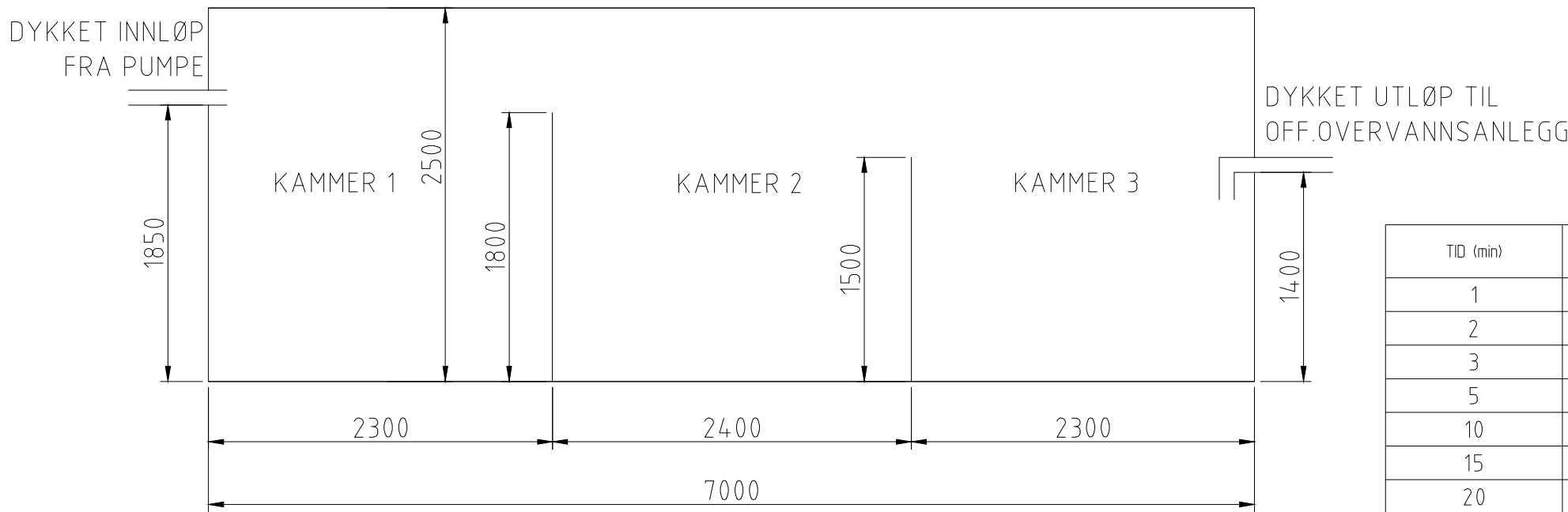
SNITT
