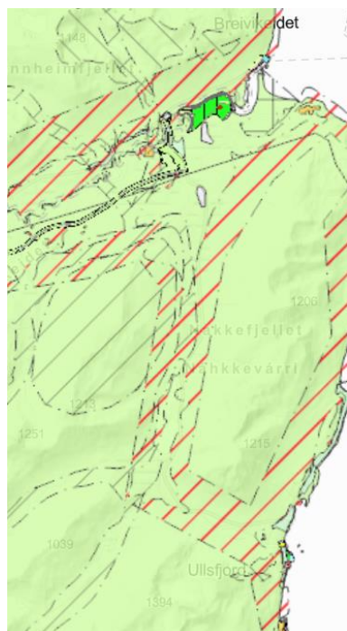
Figur 11: Faresone ras og skredfare ved Breivikeidet.
