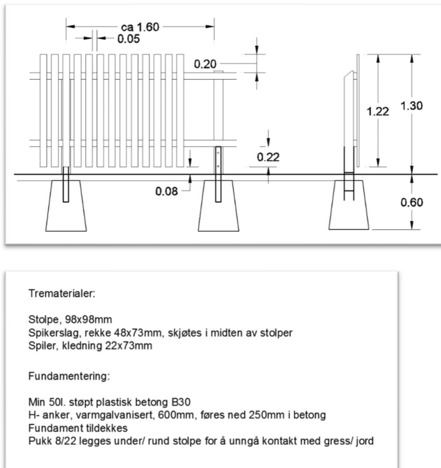
Figur 9: Eksempel for stakittgjerde
