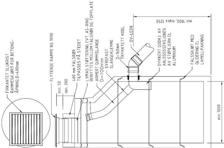
SANDFANGSKUM MED SPESIELL TOPP
