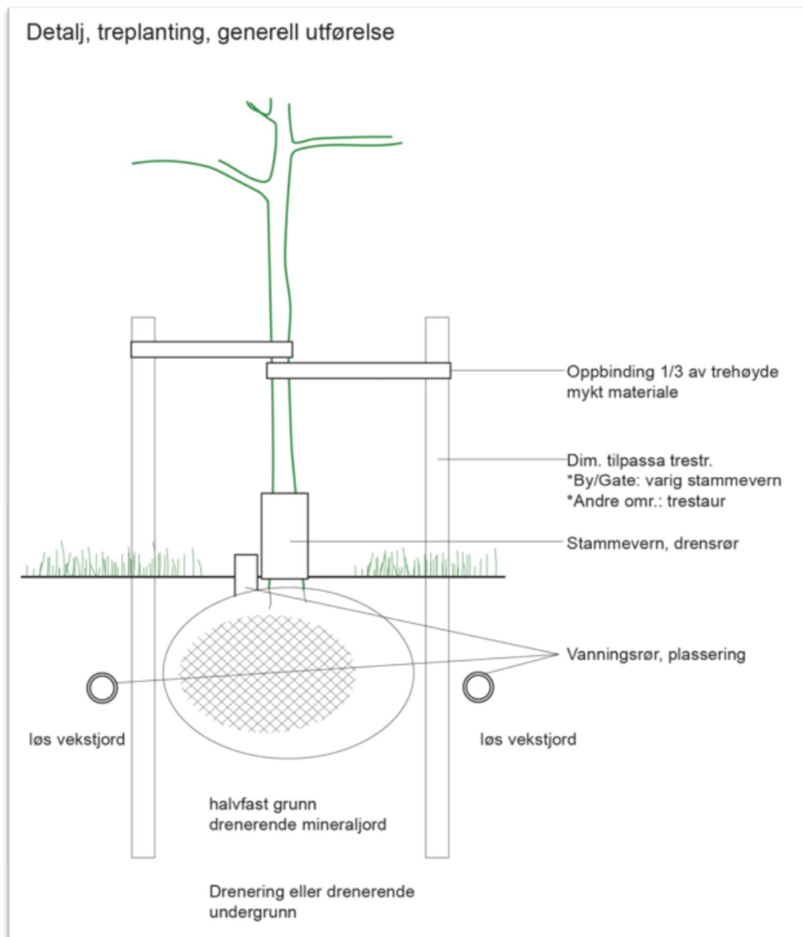
Figur 7: Prinsipp tegning for planting av trær i vegetasjonsareal
