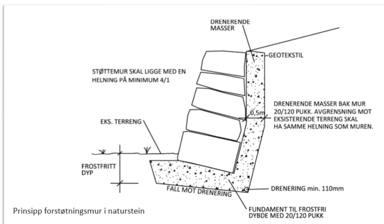
Figur 3: Eksempel for støttningsmur med lagdelt naturstein.
